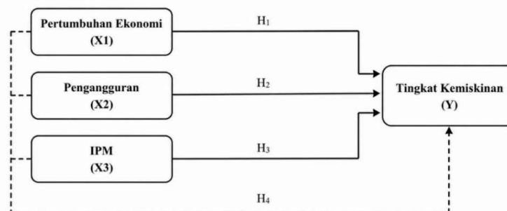
Gambar 1. Kerangka Konseptual
