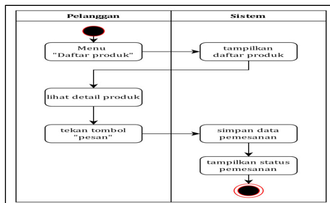
Gambar 5. Activity Diagram Pemesanan
