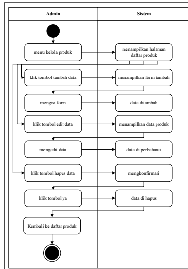
Gambar 4. Activity Diagram Kelola Produk
