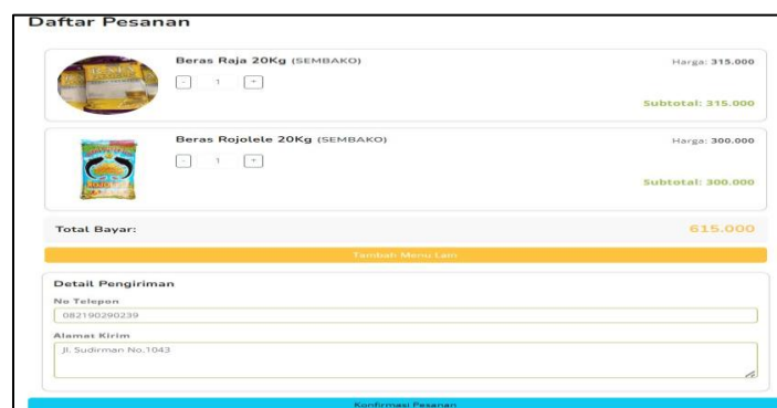
Gambar 11. Halaman Pemesanan
