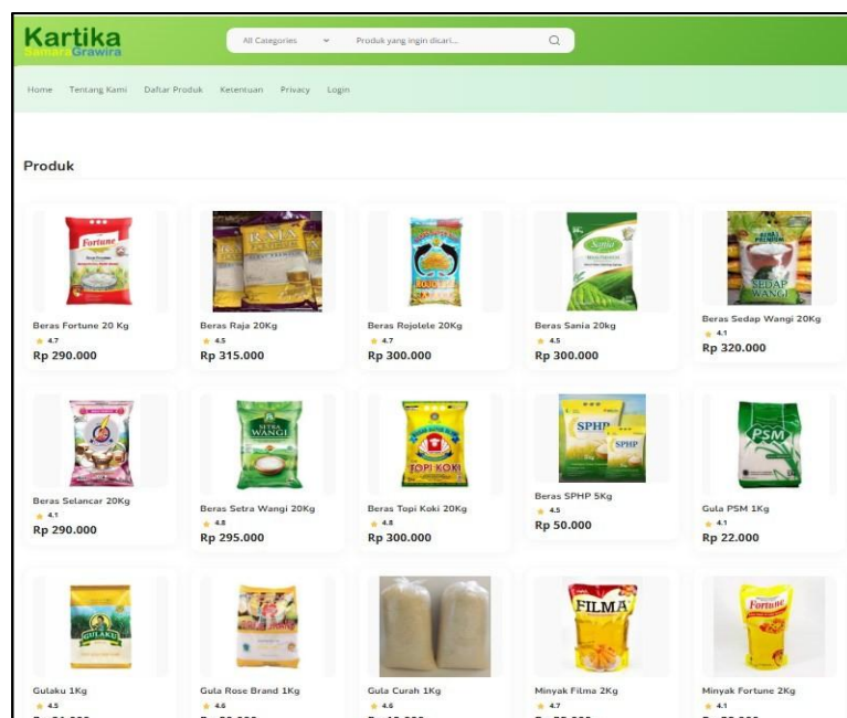
Gambar 8. Halaman Produk
