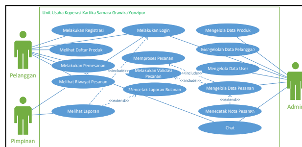
Gambar 1. Usecase Diagram Yang Diusulkan
